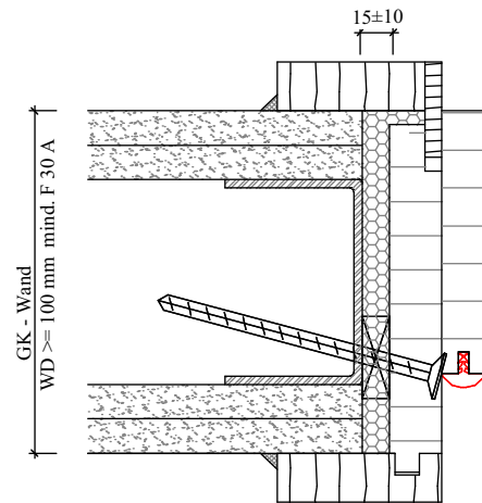
Holzumfassungszarge Einbauvariante Leichtbauwand
