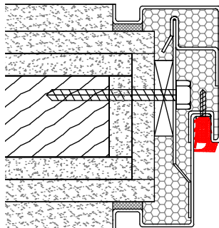
Stahleckzarge einteilig
