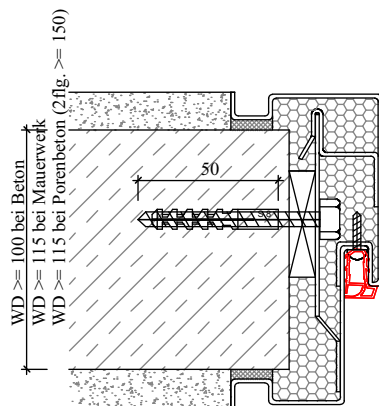
Stahlumfassungszarge einteilig
