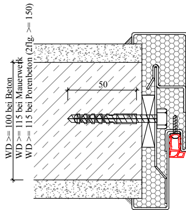
Stahlumfassungszarge zweiteilig Einbauvariante Massivwand
