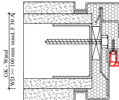
Stahlumfassungszarge einteilig
