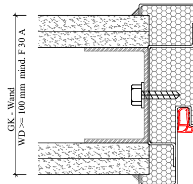
Stahlumfassungszarge einteilig
