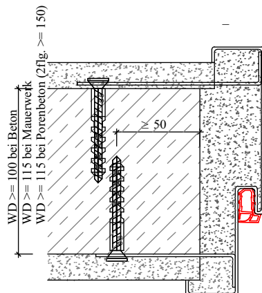
Stahlumfassungszarge einteilig
