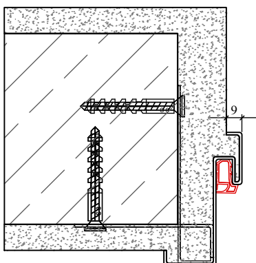
Stahleckzarge einteilig
