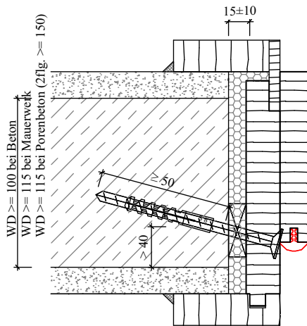
Holzumfassungszarge Einbauvariante Massivwand
